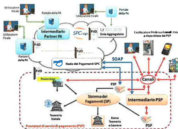
Figura 1 Schema architetturale sistema PagoPA
